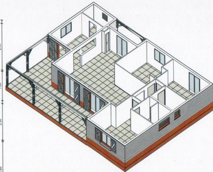
Eclaté du rez de chaussée
